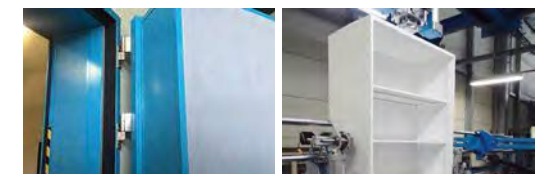
半無響室 クリーンファンユニット(空調)の試験装置「KKS-Labo」半無響室の扉500mm。 加重耐久試験装置 2016年9月に導入。災害にも強い製品の品質の維持向上のため自社での厳しいチェック体制を構築しております。
