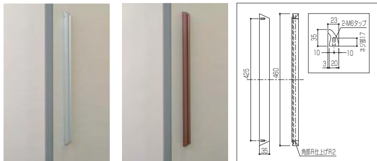
HL-01 (シルバー) HL-02 (アンバー) ●材 質：アルミ ●材 質：アルミ ●表 面：化研アルマイト処理 ●表 面：アルマイト処理
