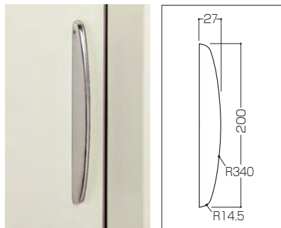
HNハンドル ●材 質：亜鉛ダイキャスト クロームメッキ仕上げ
