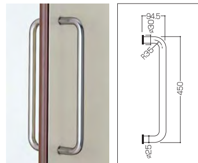
KU-01-001 ●材 質：ステンレスミラー
