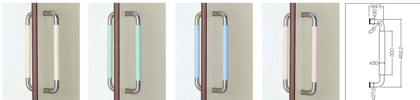
KU-01-007 (アイボリー) KU-01-008 (グリーン) KU-01-009 (ブルー) KU-01-010 (ピンク) ●材 質：本 体 ステンレスミラー 握り部 ナイロン樹脂
