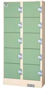
■2列5段タイプ (10人用) JH-CL10WN ¥283,920 (¥270,400) 840W×455D×1790H ●1人当り内寸: 357W×453D×318H ●質量: 83.0kg
