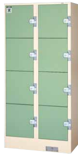
■2列4段タイプ (8人用) JH-CL08WN ¥273,105 (¥260,100) 840W×455D×1790H ●1人当り内寸: 357W×453D×398H ●質量: 76.0kg
